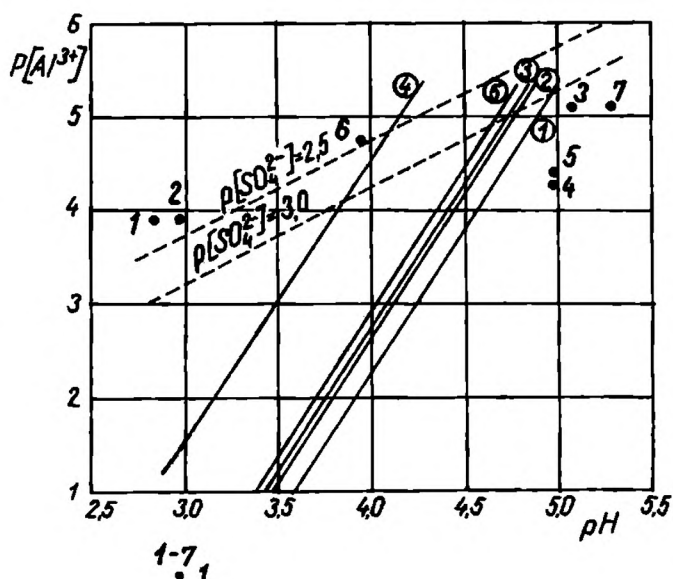
Fig. 6 Aktywność jonu glinowego w funkcji pH roztworu w równowadze z mineralami glinu (według Erikssona, 1981; van Breemen'a, 1973). Linie ciągłe: ① – amorficzny wodorotlenek glinu, ② – mikrokrystaliczny gibbsyt, ③ – gibbsyt, ④ – kaolinit p[\text{SiO}_2]=3,5 , ⑤ – halloizyt p[\text{SiO}_2]=3,5 . Linie przerywane – zasadowy siarczan glinu dla wybranych aktywności jonu siarczanowego; 1 – numery próbek wód
